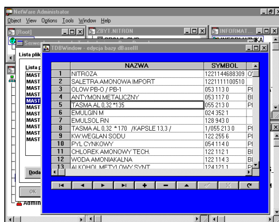
Rys. 7. Dostęp do rekordów zawartych w wyróżnionym pliku składowym bazy danych za pomocą komponentów typu TVbxControl
