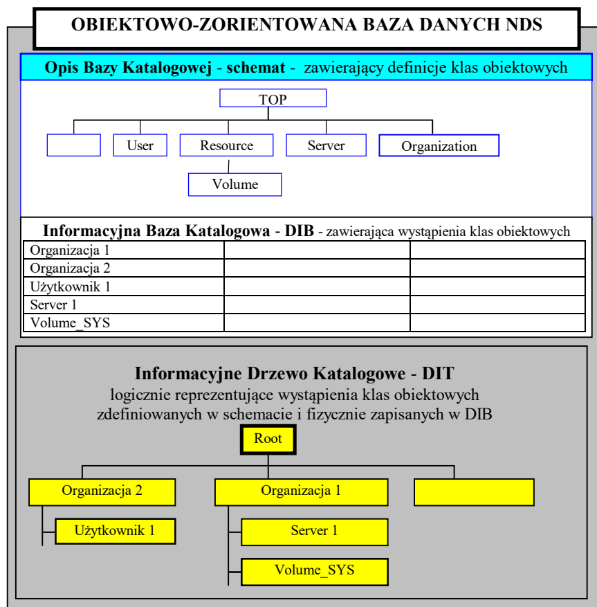
Rys. 10. Budowa obiektowo-zorientowanej bazy NDS
